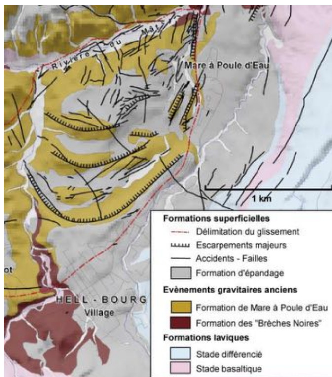
Figure 3: Carte géologique simplifiée du glissement de Mare à Poule d'Eau. Les failles ont été cartographiées à partir de leur signature morphologique. D'après Arnaud, 2005.
