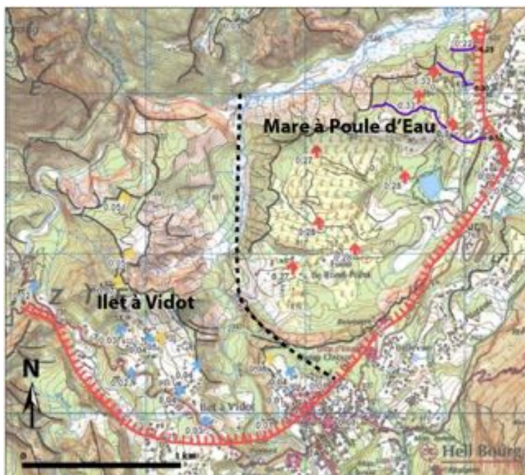
Figure 2: Limite du glissement d'Hell-Bourg (trait rouge), composé du glissement d'Illet à Vidot, à l'Ouest, et du glissement de Mare à Poule d'Eau, à l'Est. Ces deux unités de glissement se distinguent par leurs vitesses de déplacement déterminées par GPS. Les flèches indiquent le sens de déplacement et leur couleur révèle l'intensité du déplacement (de bleu à rouge pour des déplacements croissants). Les valeurs en indice correspondent aux quantités de déplacement, en mètre, mesurées entre décembre 2010 et décembre 2011. Modifié d'après Mazué et al., 2013.
